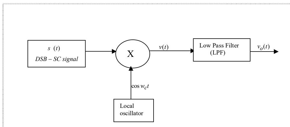
Σχήμα 7: Ανιχνευτής γινομένου για αποδιαμόρφωση DSB-SC σήματος
