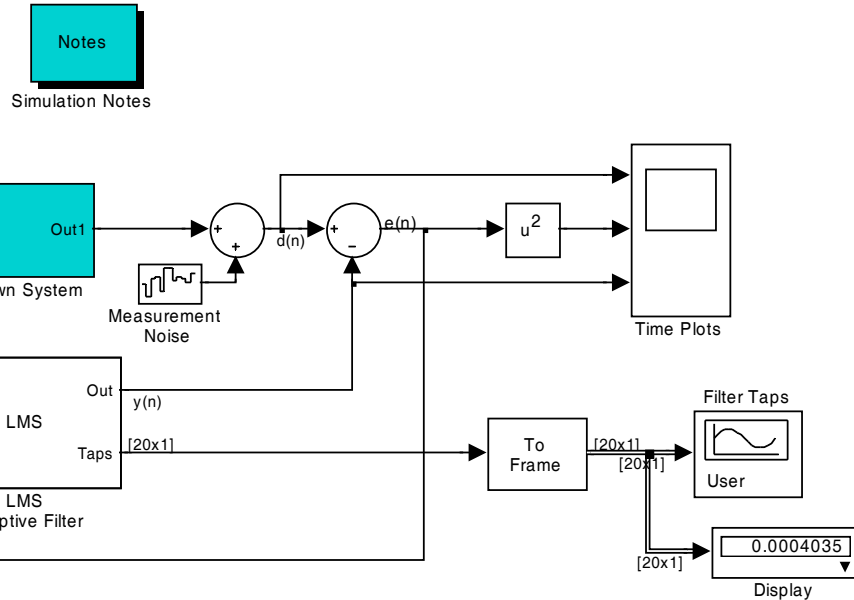
Σχήμα 2: Προσομοίωση αναγνώριση συστήματος με τη βοήθεια του SIMULINK
